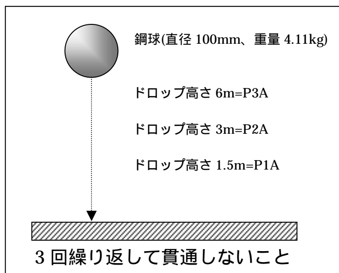
EN356 試験原理
